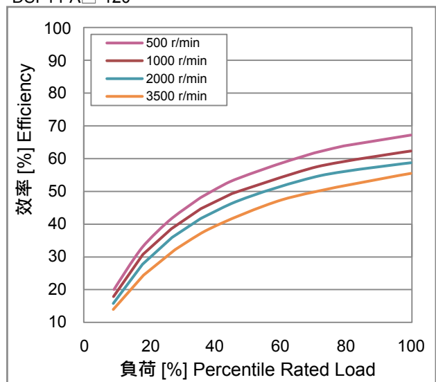
DSF14-A□-120
