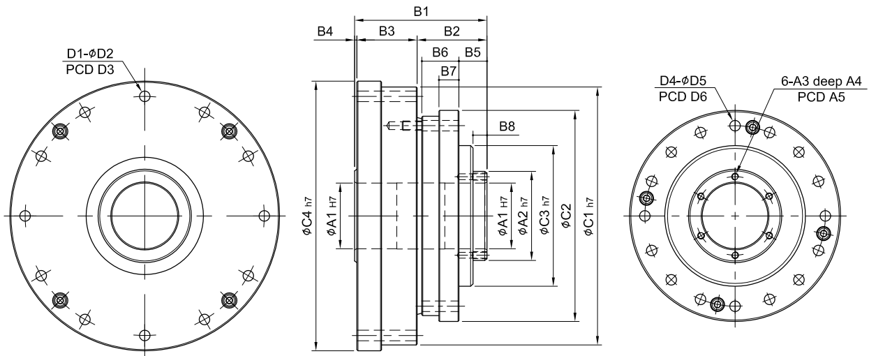
DHF14 · DHF17
