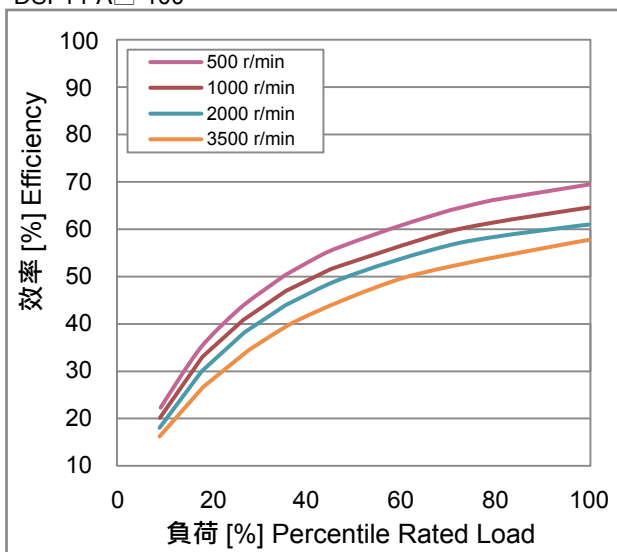
DSF14-A□-100
