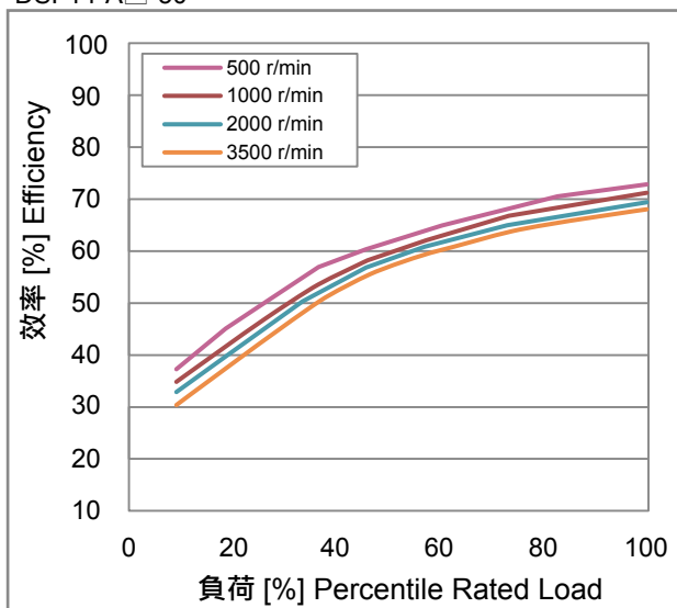
DSF14-A□-50
