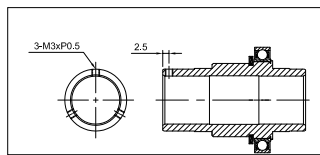
DHF14、DHF17
