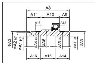
DHF20、DHF25
