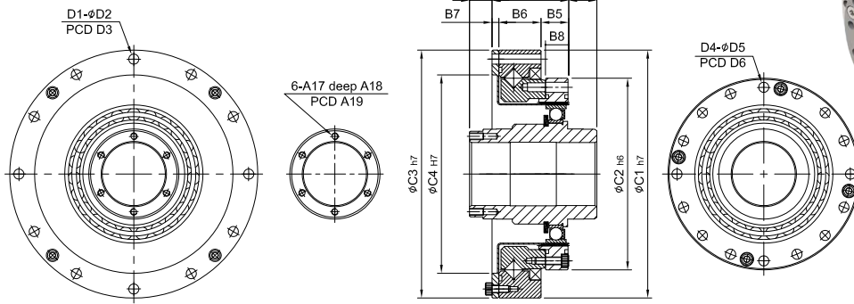
DHF20、DHF25
