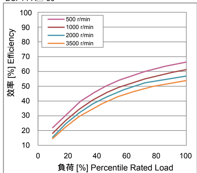
DSF14-A□-80
