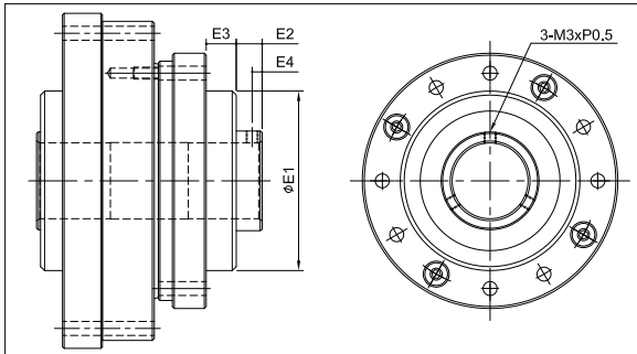
DHF14 · DHF17
